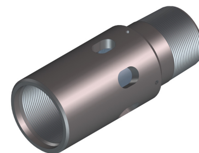
TC-FD-0350-0000 3-1/2" FILL DISC ASSEMBLY
